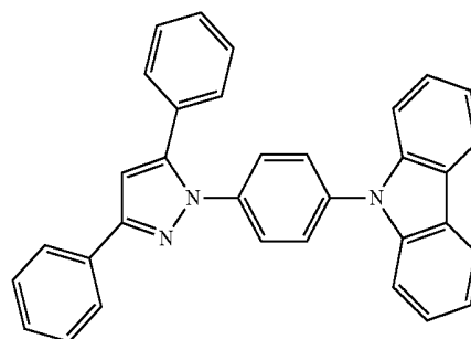
PzCz
