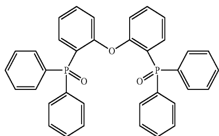
DPEPO
